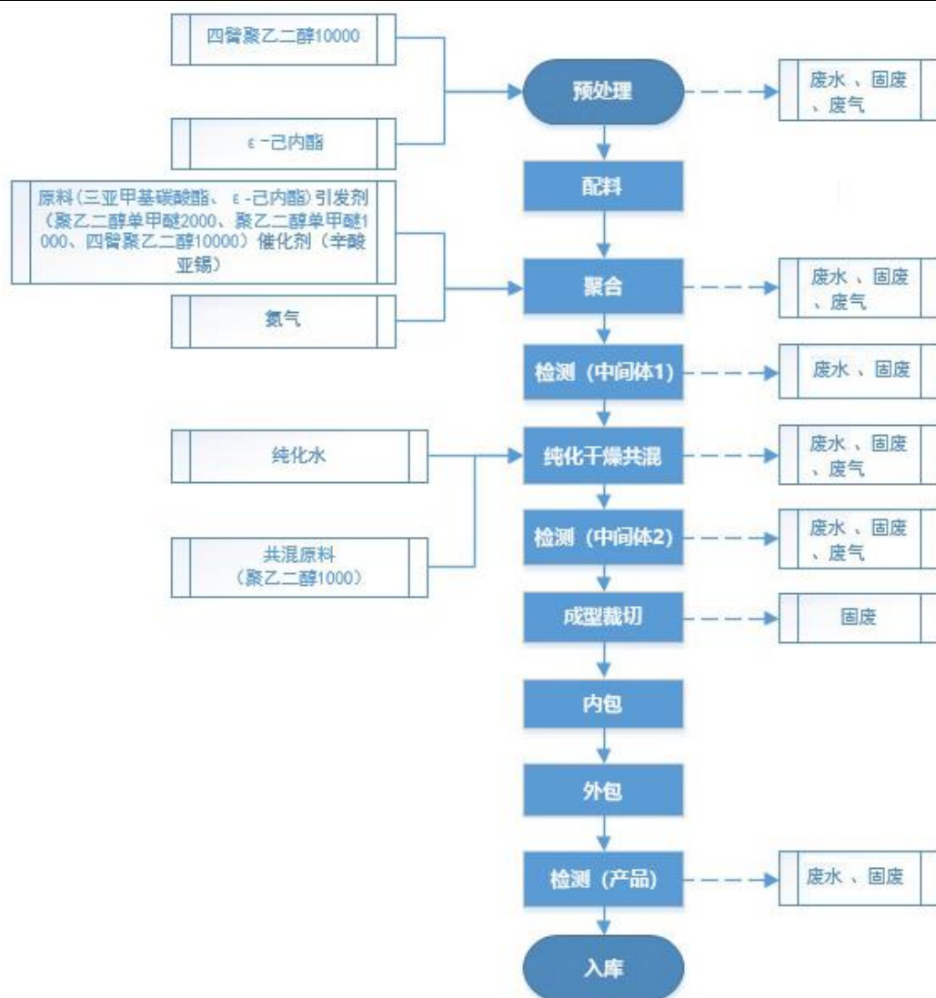
图7 本项目生产工艺流程及产污环节
