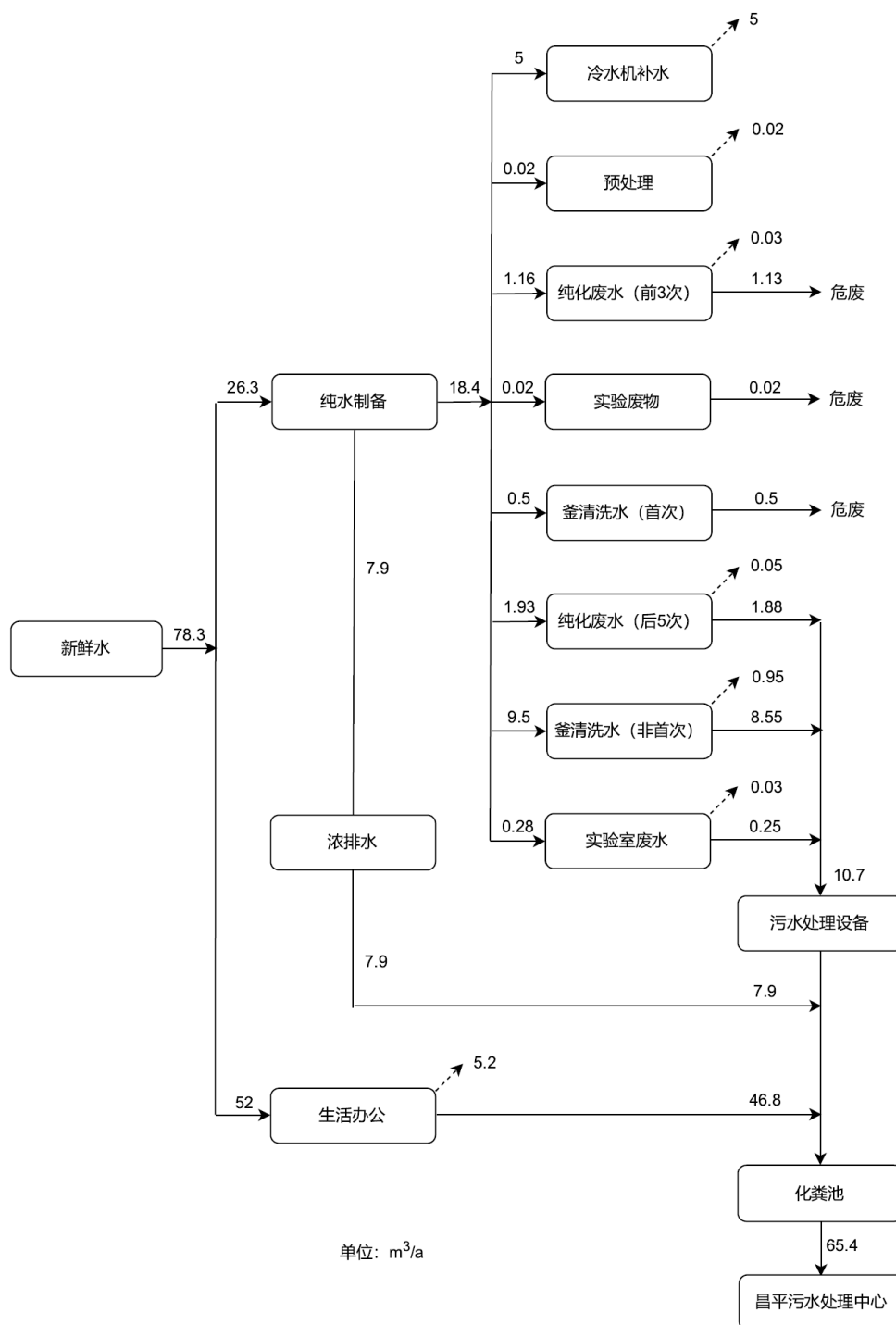
图5 本项目水平衡图
