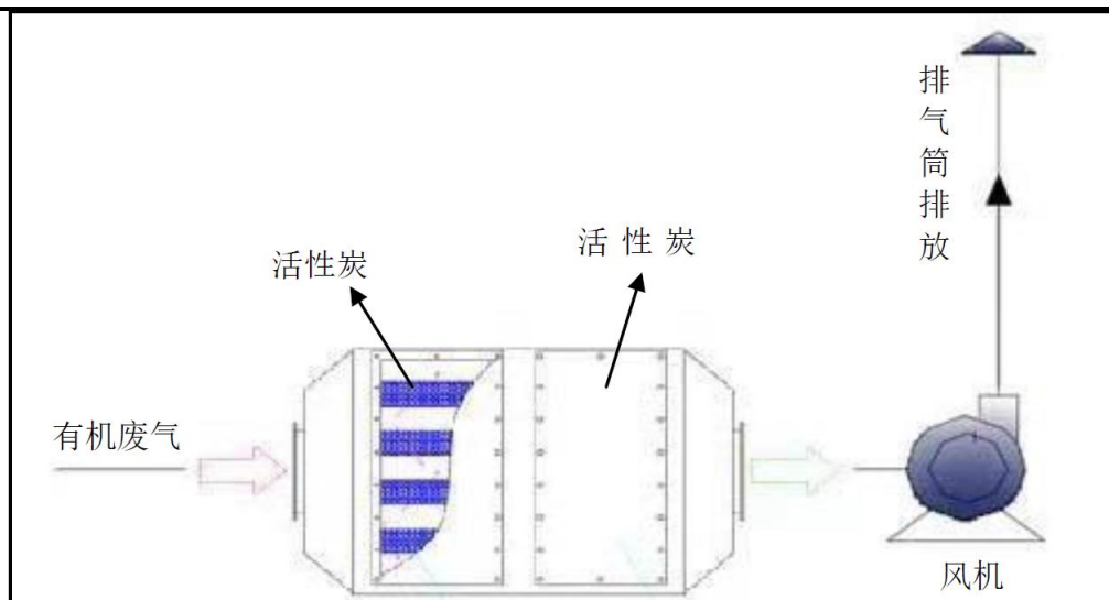
图8 活性炭吸附系统示意图
