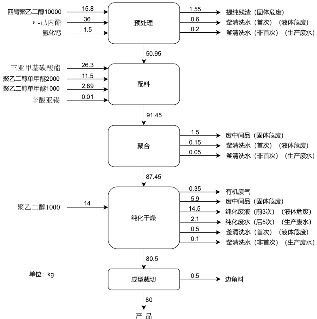
图4 本项目物料平衡图
