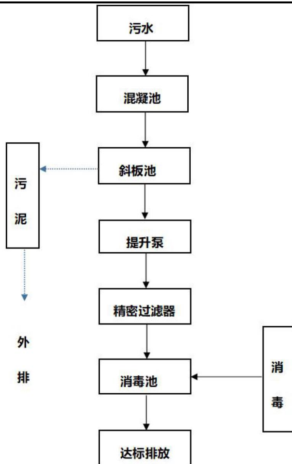
图9 污水处理工艺流程图
